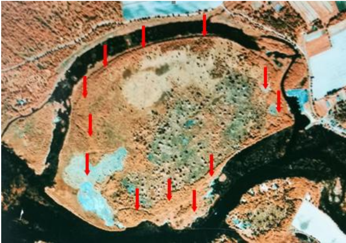
Kuva 14. Vuoden 1991 väärävärikuti Matinsaaresta. Eri ikäiset patoavat lajitysalueet osoitettu nuolilla.
