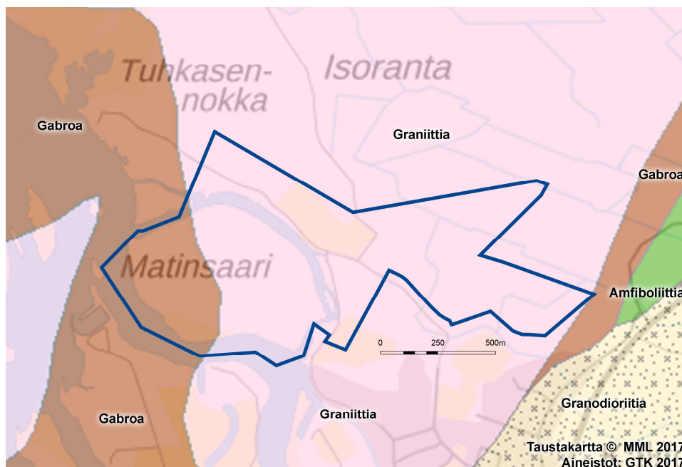
Kuva 19. Suunnittelualueen kallioperäkartta, aluerajaus on esitetty tummansinisellä (lähde: GTK 2017)
