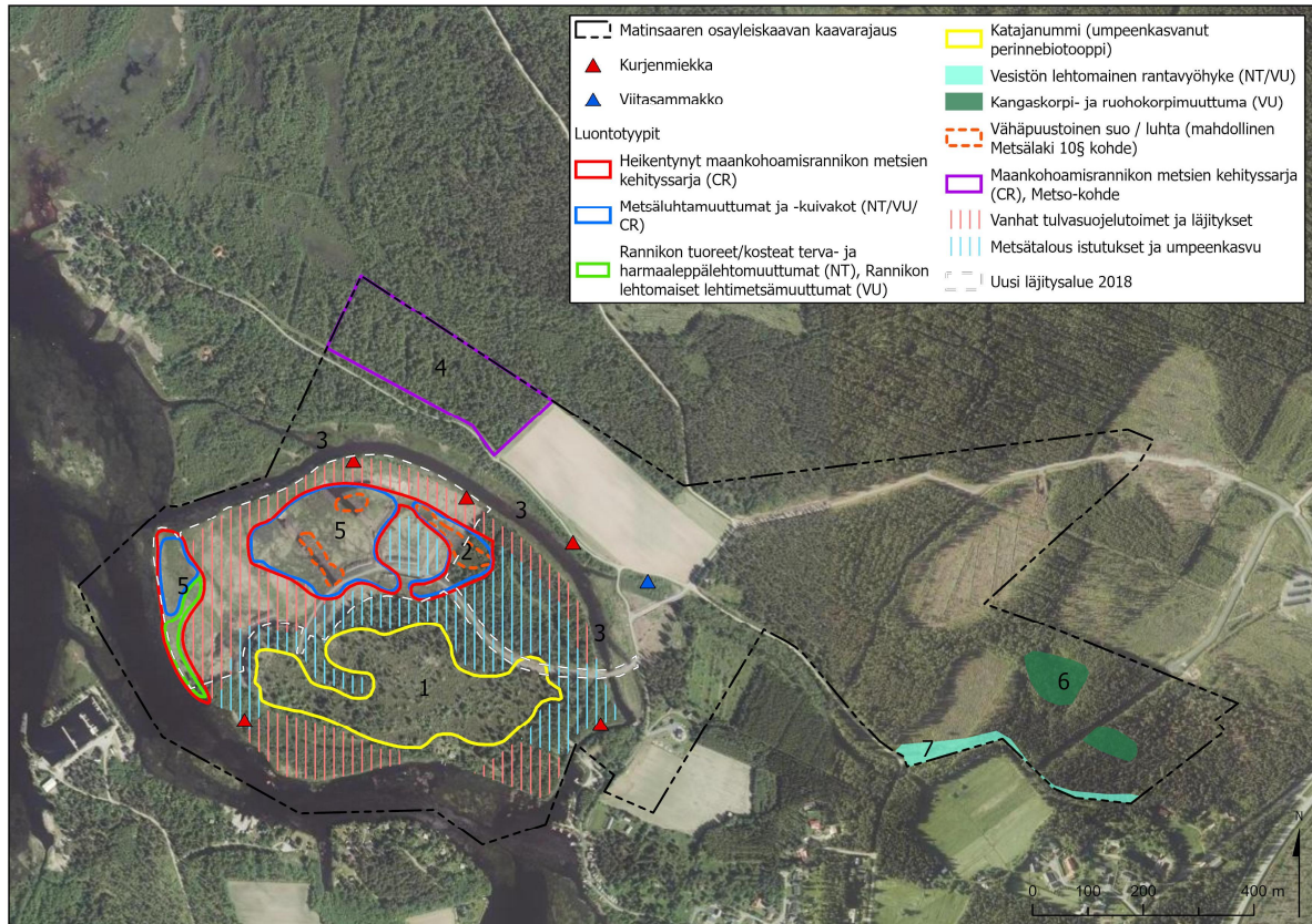
Kuva 18. Kaava-alueen luontoarvot suunnittelualueelle 2016-2020 tehtyjen kartoituskäytien mukaisesti. Numerot viittaavat tekstiin.
