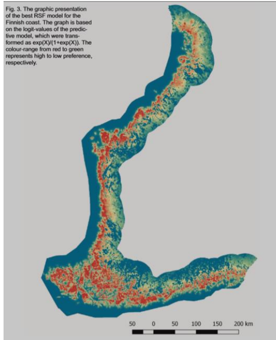
Kuva 1. RSF-mallin mukaan esiäikeisten merikotkien habitaattivalinta (suosii punaista, välttää sinistä) ja sen perusteella arvioitu lentoaktiivisuus rakennetuilla ja suunnitelluilla tuulivoima-alueilla (Tikkanen ym. 2018).
